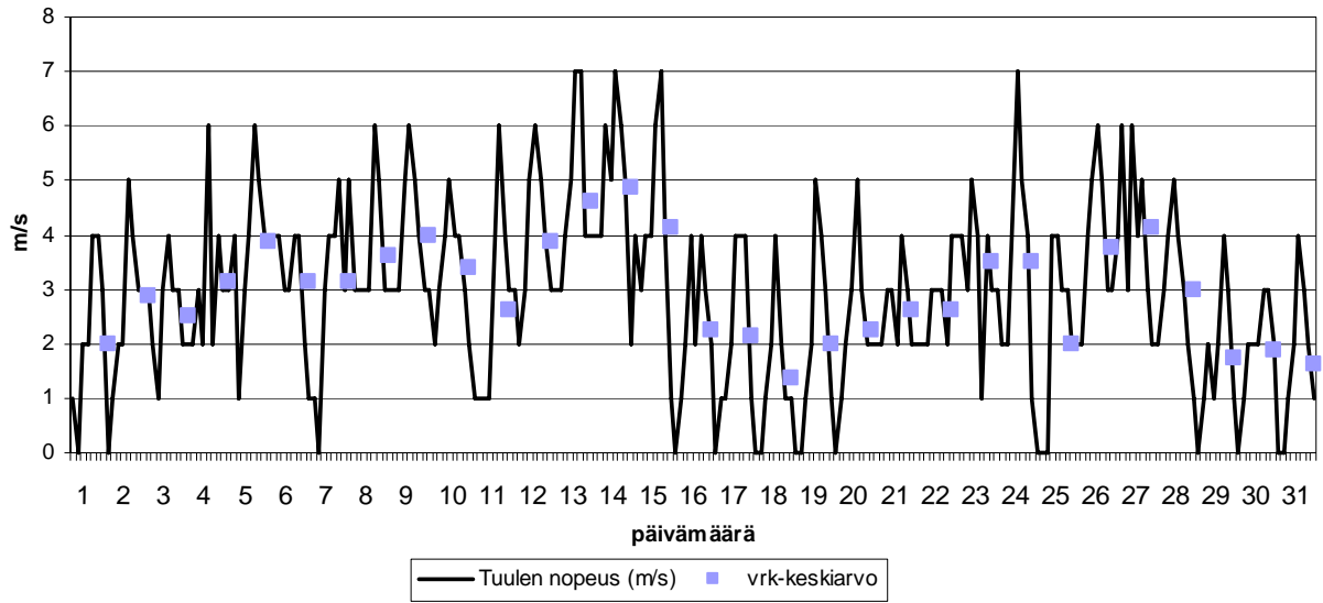
KUVA 13. Tuulen nopeus (m/s) 8 kpl/vrk sekä päivittäiset keskiarvot 1.5.-31.5.2009.
