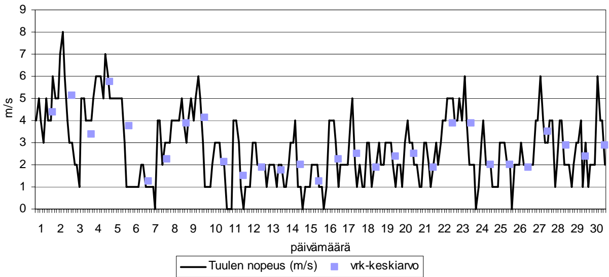
KUVA 14. Tuulen nopeus (m/s) 8 kpl/vrk sekä päivittäiset keskiarvot 1.9.-30.9.2009.
